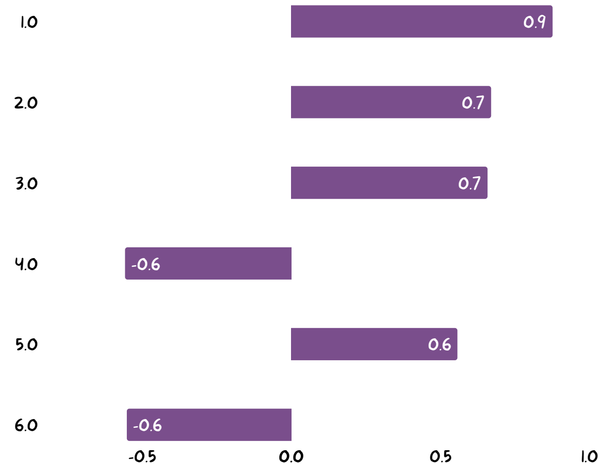
Loading terbesar PC2 (18,97%)
